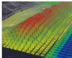
●メッシュ土量計算
