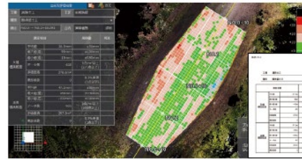
●出来形ヒートマップ
