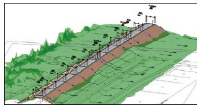
●三次元設計データ作成
